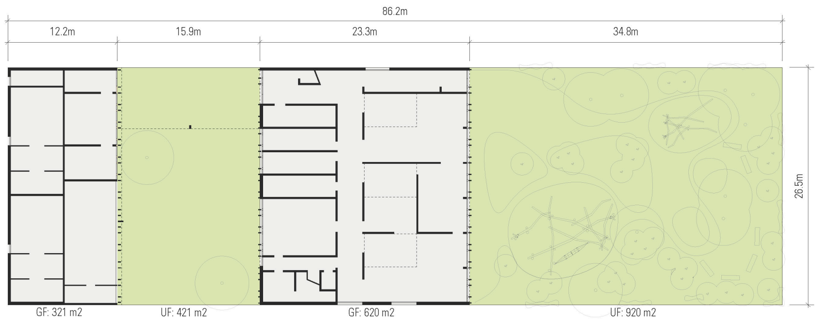
Grundriss Erdgeschoss Stand Wettbewerb 06.08.2013
