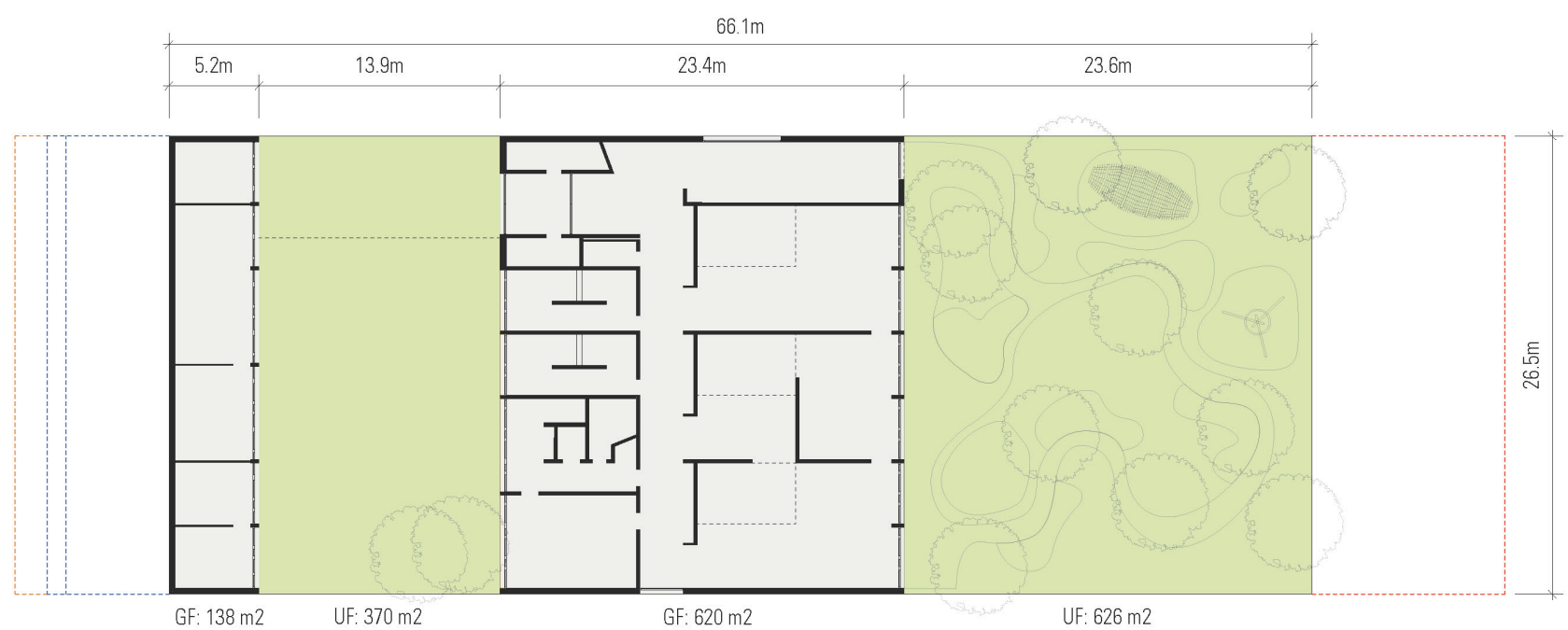
Grundriss Erdgeschoss Stand Bauprojekt 25.02.2014
