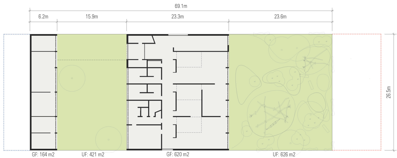
Grundriss Erdgeschoss Stand Vorprojekt 09.12.2013
